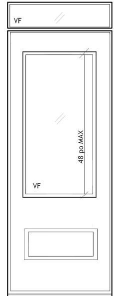
Porte simple Panneaux décoratifs en RELIEF (1 ou 2 sections) Vitrage FIXE 36 po ou 48 po maximum Imposte 1 ou 2 section
