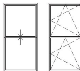
OU Fenêtre à auvent ou à battant ou oscillo-battante 2 vantaux avec meneau horizontal
