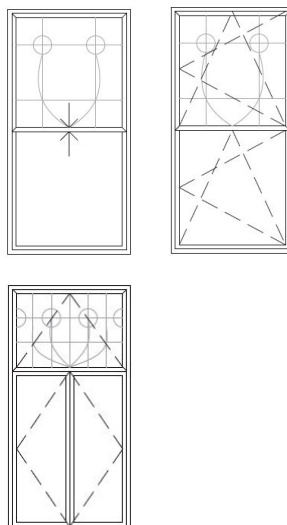
Fenêtre à auvent ou à battant ou oscillo-battante 2 vantaux avec meneau horizontal Vitreaux dans la portion du haut
