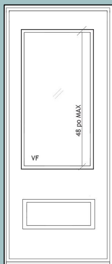
Porte simple Panneau décoratif en RELIEF (1 ou 2 rangées) Vitrage FIXE 48 po maximum
