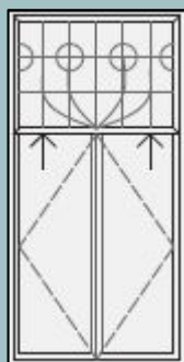
Fenêtre à guillotine \frac{1}{3} - \frac{2}{3} avec battants (ou à crémonne) 2 vantaux Vitraux dans la portion du haut
