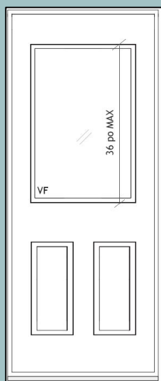
Porte simple Panneaux décoratifs en RELIEF (2 sections) Vitrage FIXE 36 po maximum
