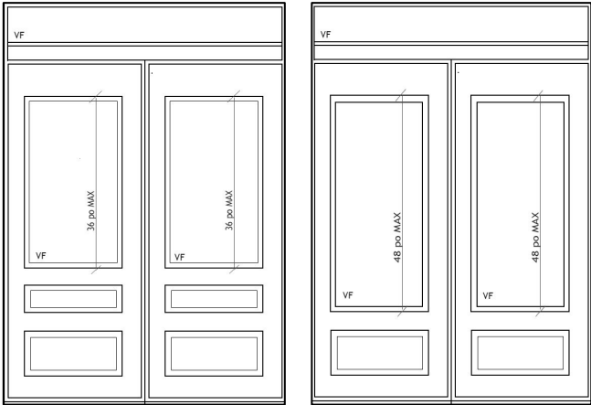
Porte double Panneaux décoratifs en RELIEF 1 section, rang simple ou double Vitrage FIXE 36 po ou 48 po maximum imposte 1 section
