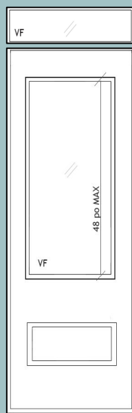
Porte simple Panneau décoratif en RELIEF Vitrage FIXE 48 po maximum Imposte 1 section
