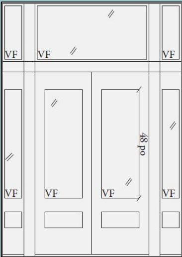
Porte double avec impostes latéraux Panneaux décoratifs en RELIEF Vitrage 48 po Impostes en plusieurs sections
